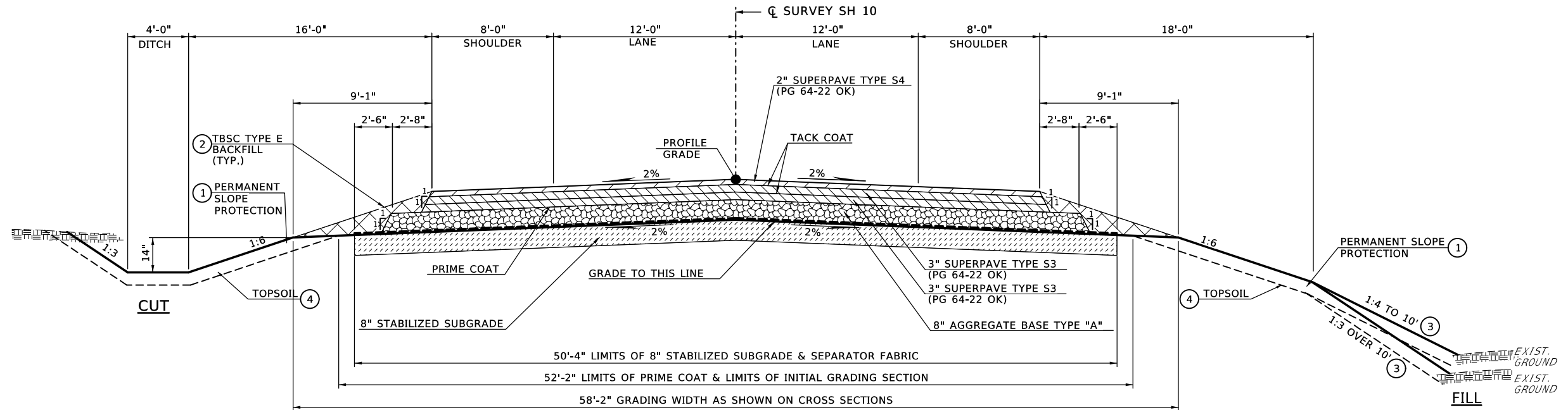
1 SH 10 TYPICAL SECTION STA. 1433+40.00 TO STA. 1436+64.15 N.T.S. STA. 1439+34.65 TO STA. 1443+30.00
