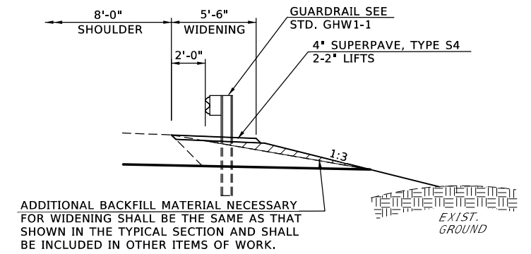
GUARDRAIL DETAIL N.T.S. STA. 1434+71.00 TO STA. 1436+64.75 RT. STA. 1434+33.50 TO STA. 1436+64.75 LT.(OPPOSITE HAND) STA. 1439+34.05 TO STA. 1440+77.80 RT. STA. 1439+34.05 TO STA. 1442+52.80 LT.(OPPOSITE HAND)
