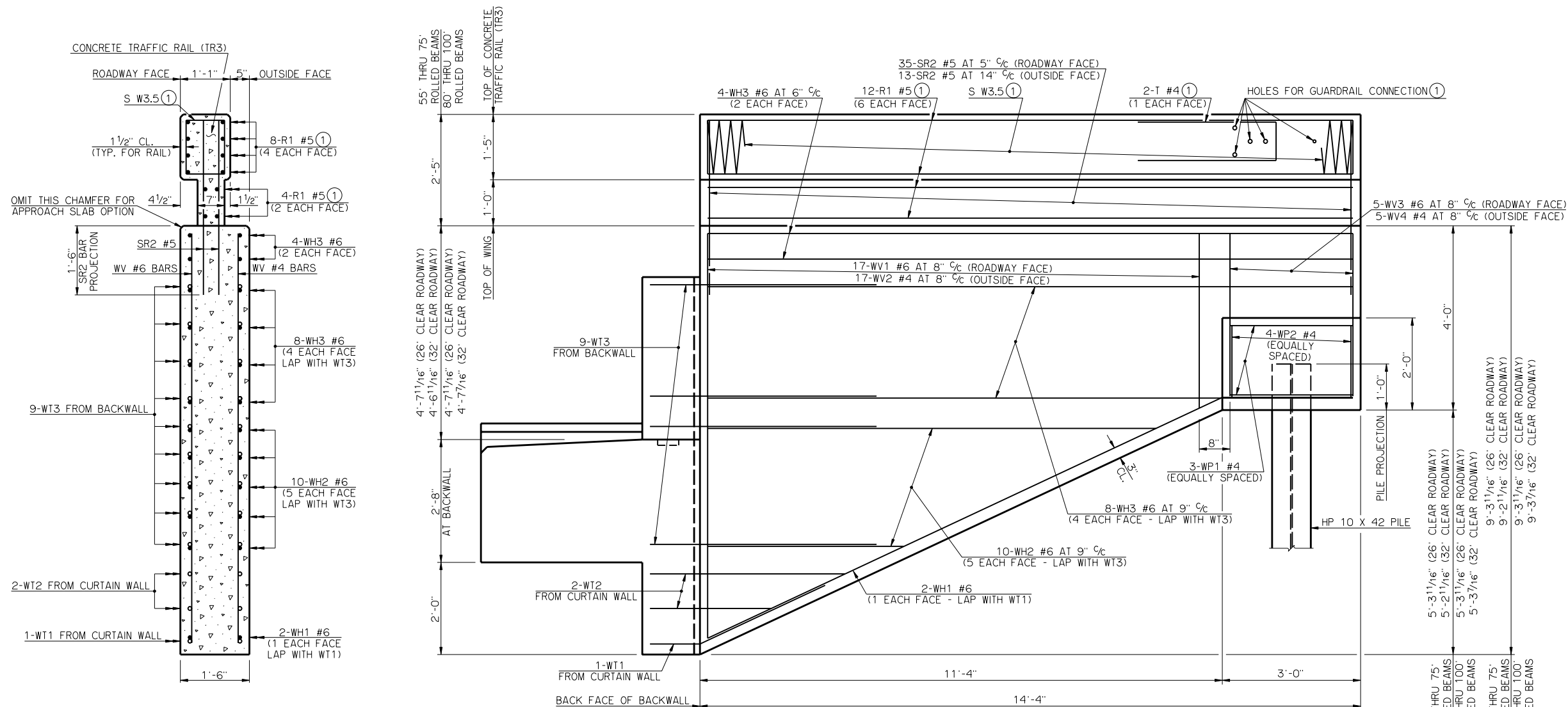
ELEVATION
