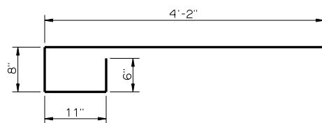
UD1 #4 X 6'-3"
